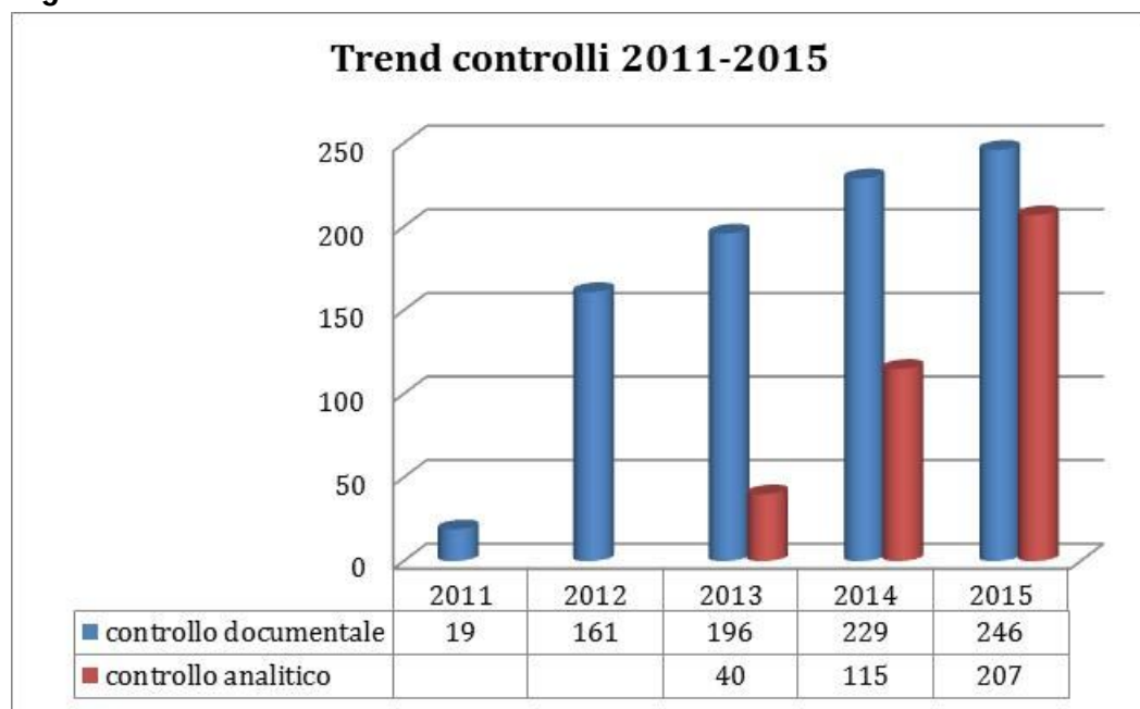
Figura 9 – Trend controlli-Anni 2011-2015
